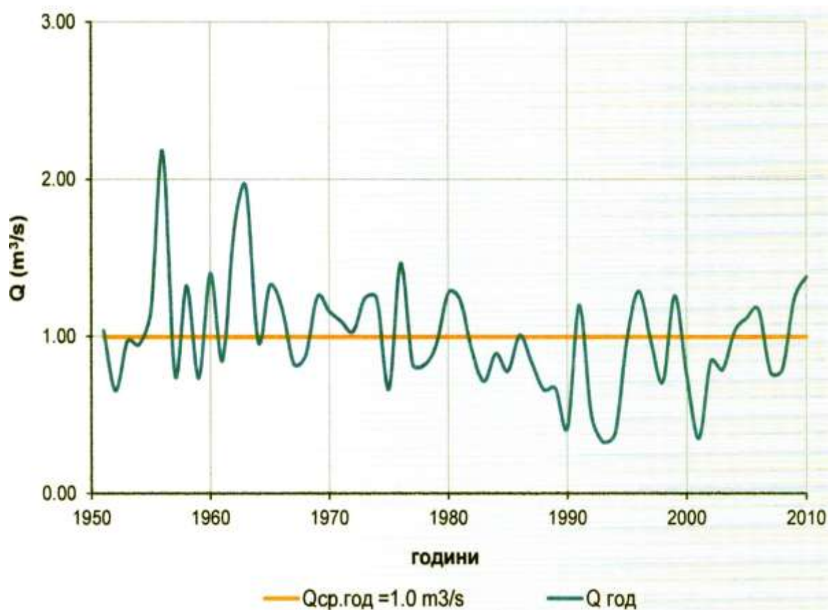
График 4. Средно месечни протеци на р. Злетовска/ м.м Кнежево (54,6 km 2 )
