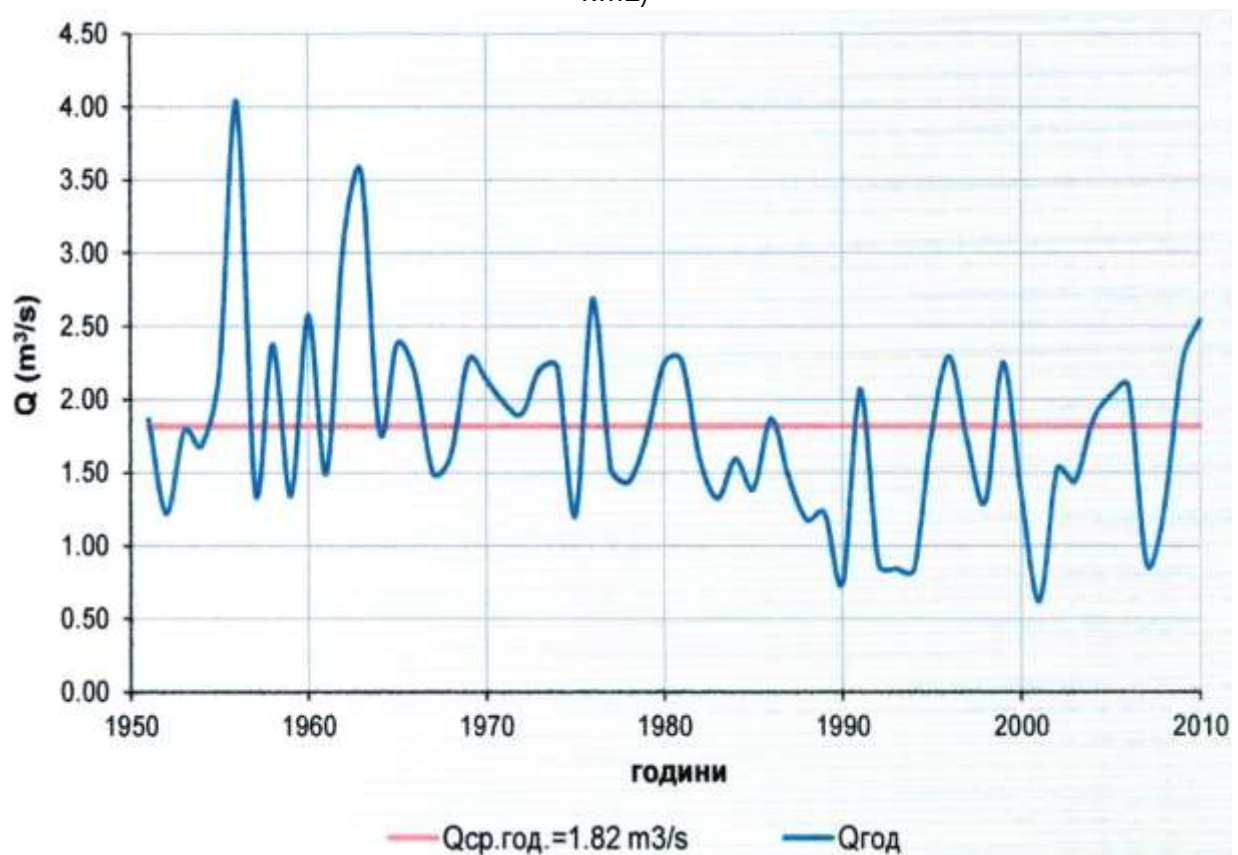
График 6. Средно месечни протечи на р. Злетовска/ м.м Зафат на Пробиштип (109,2 km 2 )
