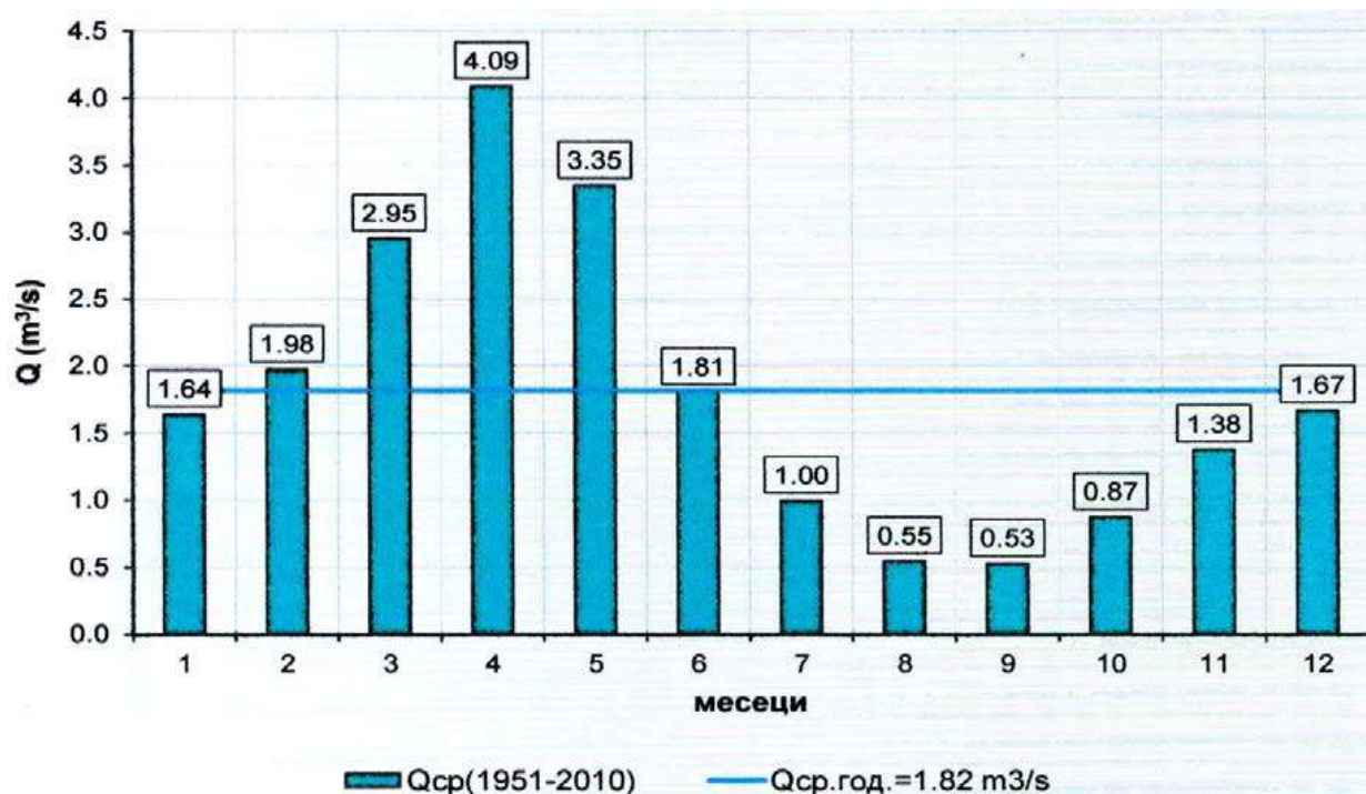
График 5. Средно месечни протечи на р. Злетовска/ м.м Зафат на Пробиштип (109,2 km 2 )
