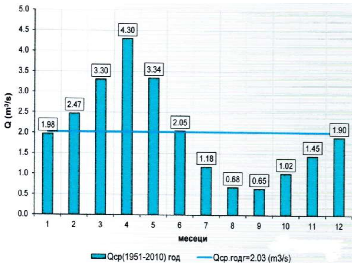
График 1. Средно месечни протечи на р. Злетовска/ В.Ст Злетово (172 km 2 )
