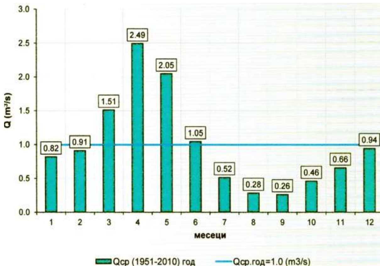
График 3. Средно месечни протеци на р. Злетовска/ м.м Кнежево (54,6 km 2 )
